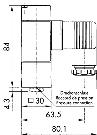
Stecker / Connecteur / Plug DIN 43650-A
