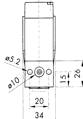
Stecker / Connecteur / Plug DIN 43650-A (GL)
