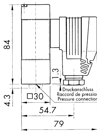
Stecker / Connecteur / Plug DIN 43650-A (GL)
