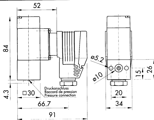
Stecker / Connecteur / Plug DIN 43650-A (GL) (Zubehör 59 / Accessoire 59 / Accessory 59)
