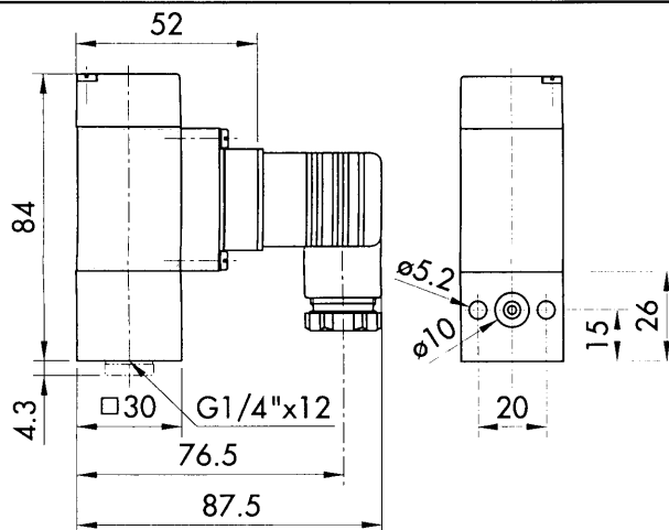
Stecker / Connecteur / Plug DIN 43650-A (Zubehör 58 / Accessoire 58 / Accessory 58)
