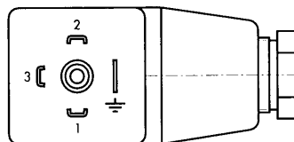
DIN 43650-A (GL)
